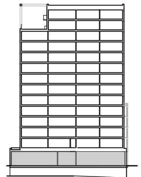
SEKTION SKALA 1:500
